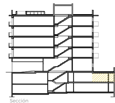
Sección
